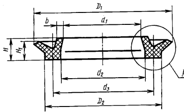
Исполнение 1 I Исполнение 2
